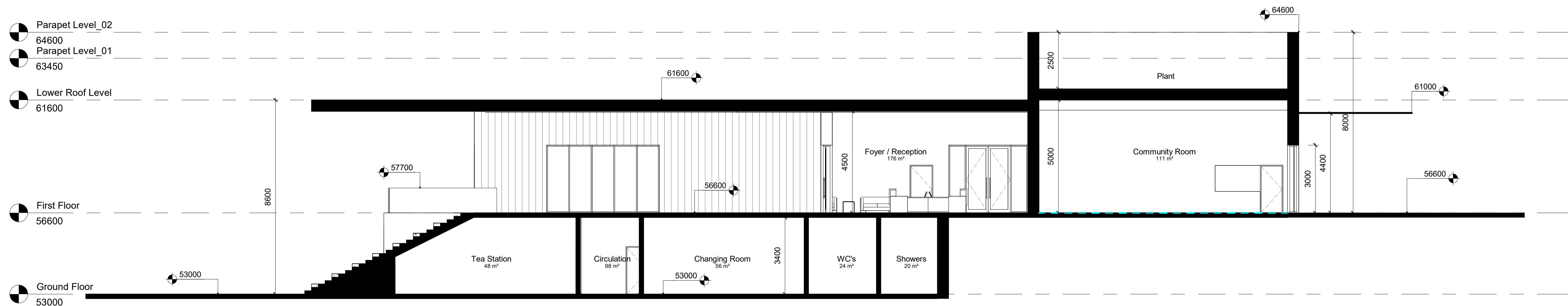
Section AA 1 : 100
